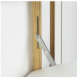
Klappwinkel kann durch einsetzen mehrere Magneten variiert werden / Folding angle can be varied by using several magnets
